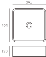
CS-0094 Size: L x W x H 395X395X120MM N. W: 13.4KG
