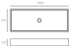
CS-0098 Size: L x W x H 1005X395X120MM N. W: 30.5KG
