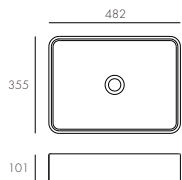
CS-0080 Size: L x W x H 482X355X101MM N. W: 12.5KG
