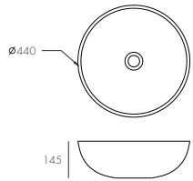
CS-0053 Size: L x H 440X145MM N. W: 7.6KG
