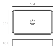
CS-0081 Size: L x W x H 584X355X101MM N. W: 15KG
