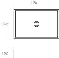
CS-0116 Size: L x W x H 496X396X120MM N. W: 18KG
