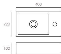
CS-0018 Size: L x W x H 400X220X100MM N. W: 6.5KG
