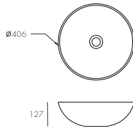
CS-0083 Size: L x H 406X127MM N. W: 7.KG
