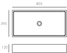
CS-0097 Size: L x W x H 805X395X120MM N. W: 29KG
