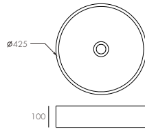
CS-0003 Size: D x H 425X100MM N. W: 12KG
