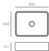
CS-0079 Size: L x W x H 406X304X101MM N. W: 9KG
