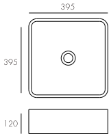
CS-0108 Size: L x W x H 395X395X120MM N. W: 12.5KG
