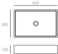
CS-0096 Size: L x W x H 605X395X120MM N. W: 22KG
