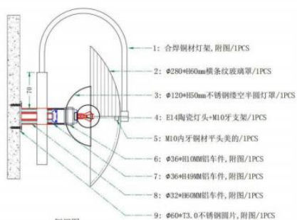
側視圖
