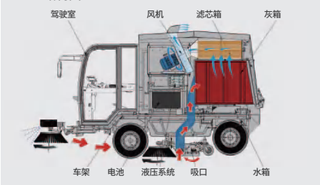
S2000结构图
